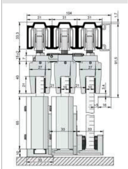
HELM 73, Deckenmontage mit HELM Untere Führung spielfrei und HELM Untere Führung zweigeteilt
