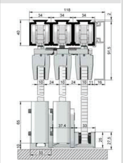
HELM 140, Deckenmontage mit HELM Untere Führung spielfrei und HELM Untere Führung zweigeteilt
