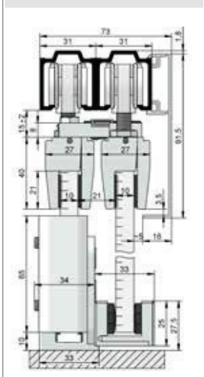
HELM 73, Deckenmontage mit HELM Untere Führung spielfrei und HELM Untere Führung zweigeteilt
