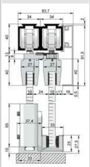
HELM 140, Deckenmontage mit HELM Untere Führung spielfrei und HELM Untere Führung zweigeteilt
